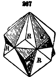
Hematite.
